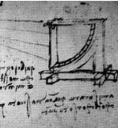
Původní náčres L. da Vinciho kyvadlového anemometru (přístroj na měření rychlosti větru) a model vyrobený v současnosti.
